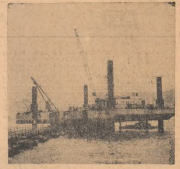
Pe șantierul hidrocentralei Porțile de Fier, Cu ajutorul platformei plutitoare, se con- struiesc pilonii de la Porți omonia Foto: AGERPRES
