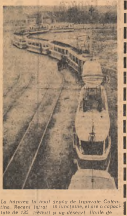
La intrarea în noul depou de tramvaie Colentina. Recent intrat în funcțiune, el are o capacitate de 135 trenuri și va deservi liniile de tramvaie 1, 4 și 21
