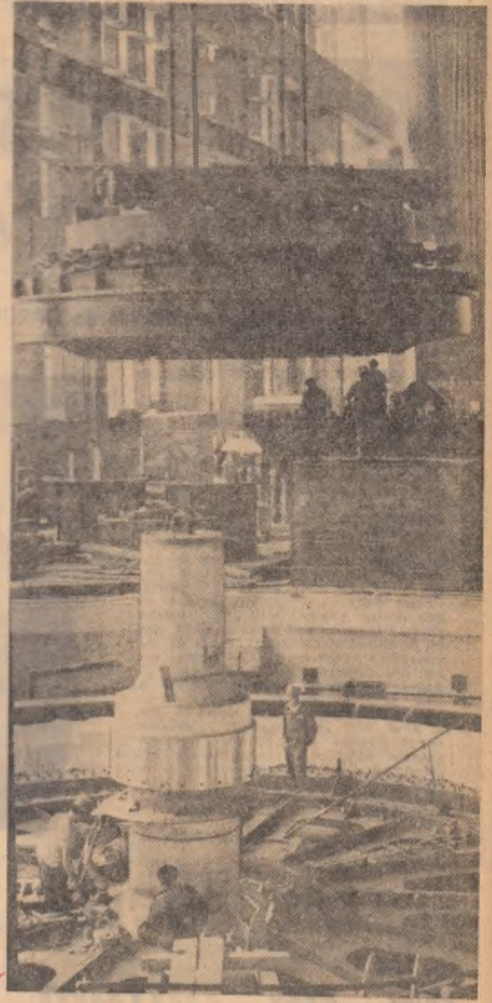
Montarea generatoarelor la hidrocentrala de la Porțile de Fier — numai rotorul cântărește 650 t.
