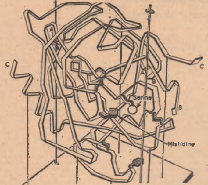
Imaginea reprezintă structura unei molecule de chimotropism. După cum se vede cele trei lanțuri separate A, B și C sunt unite între ele prin punți de bisulfid. Cei doi aminoacizi, histidina și serina, determină acuitatea catalitică a enzimei.
