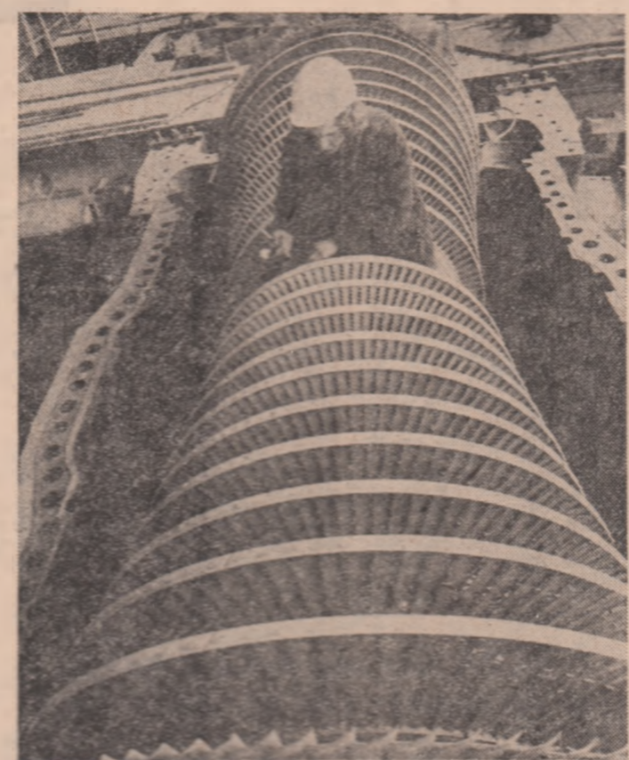
R. P. POLONĂ — Aspect de pe șantierul centralei electrice KOZIENICE, unde până în prezent au fost puse în funcțiune opt grupuri cu o putere totală de 1.600 MW, urmind ca în continuare să mai fie puse în funcțiune încă două grupuri de câte 500 MW
