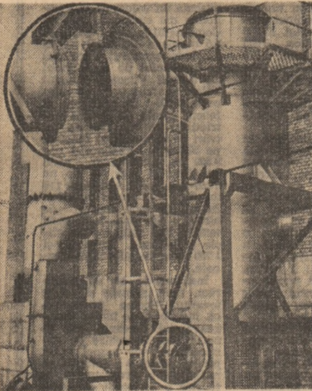
Așa arată unul din cele două recuperatoare de căldură proiectate (incomplet) de I.P.C.M. P-7 precum și o reprezentare lămurită a unui nod, proiectantului mai este dator și cu alte componente...
