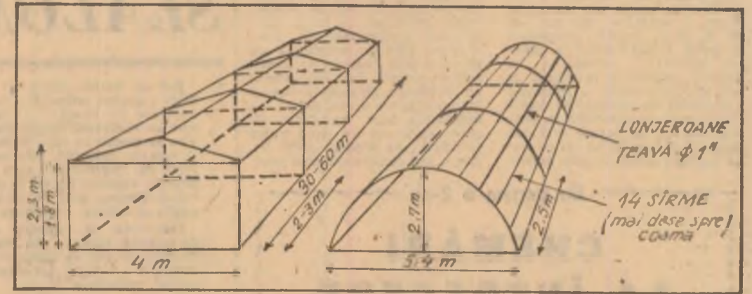
Solar in 2 pante, cu structura de rezistență din lemn (stînga). Solar tunel, cu structura de rezistență din arc de țeava (dreapta)
