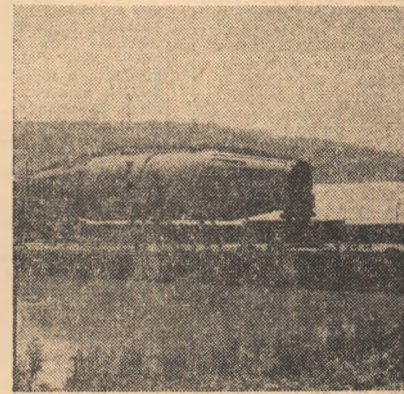
Transportul pe uscat și pe apă al celui mai greu utilaj tehnologic realizat pentru chimia națională, reactorul de 210 t pentru C.P. Mîdia.
