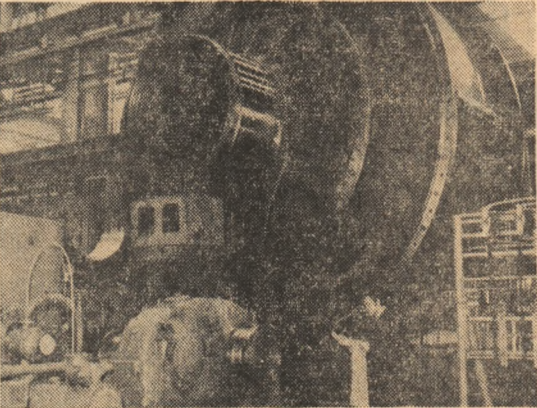
Instalații de mare capacitate și complexitate destinate industriei de prelucrare a minereului. Concepute și realizate la Întreprinderea de mașini grele București, unitate care și-a marșit continuu gama de utilaje destinate industriei noastre și pentru export
