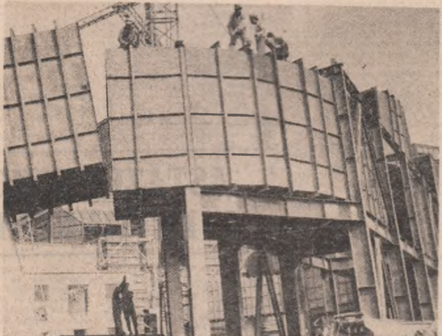
Montajul — proba de maturitate a colectivului. Cu atât mai mult cu cât fotoreporterul surprinde echipa condusă de către maestrul Florea Cătruna care lucrează la montarea canalelor de gaze arse la cosul de fum al cazanului numărul 4 — cel mai important obiectiv al acestor zile.
