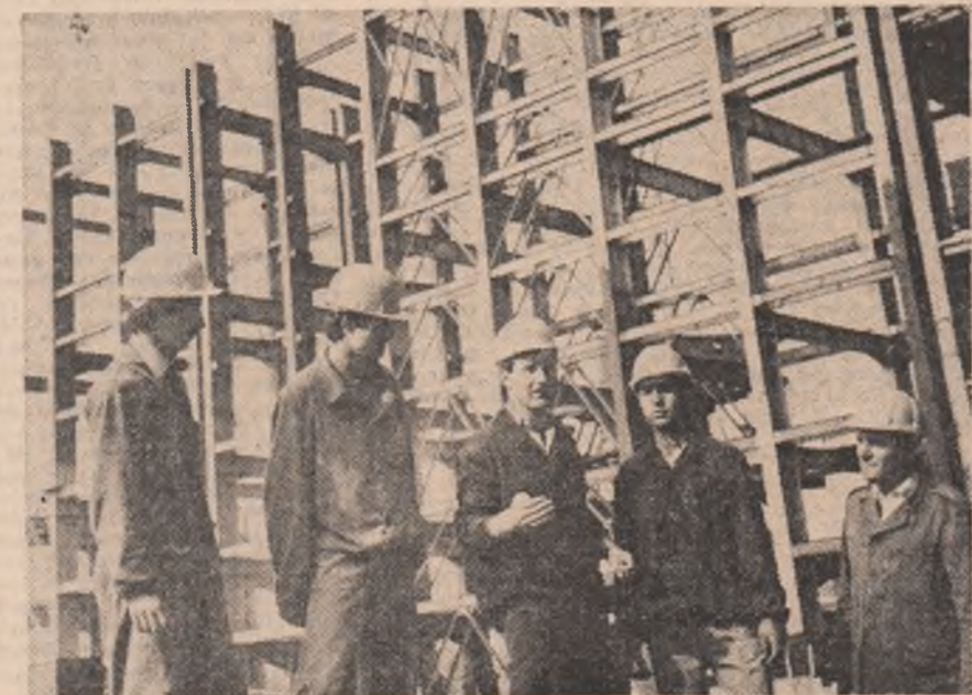
Calitatea este o cerință prioritară pentru toate activitățile de șantier. O lucrare cum este și cea din imagine — centrarea și montarea ansamblului motor-rotor care va pune în funcțiune ventilatorul de gaze arse — presupune profesionalism dar și exigență și, evident, responsabilitate. Calități pe care le întrunește pe de-a-nregul echipa condusă de maestrul Gheorghe Ababei.
