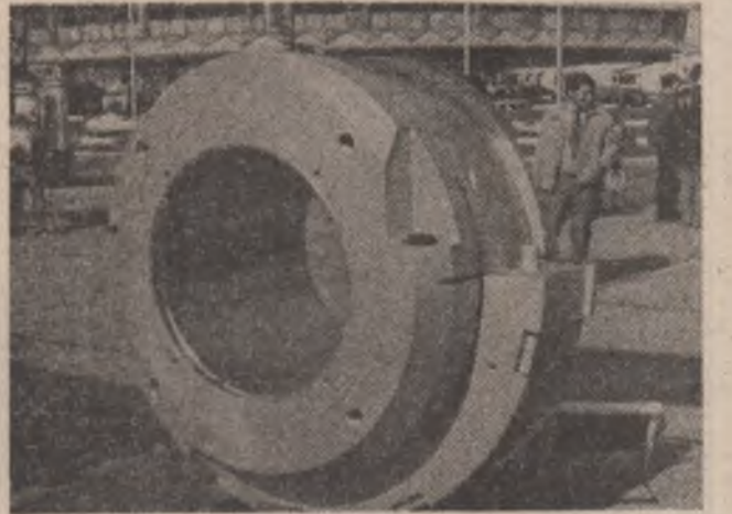
LAGĂR RADIAL pentru grup de 700 MW, utilizat în centralele nucleare — reprezintă o reușită de maximă importanță pentru sectorul energetic, probînd înaltul potențial al industriei românești. Acest lagăr este pe de altă parte o expresie „materializată” a bunelor relații de colaborare cu firme de prestigiu de peste hotare, fiind rod al cooperării Întreprinderii de Mașini Grele București, cu General Electric — S.U.A. „Perechea” lagărului din imagine, expus în stăndurile Romenergo, poate fi văzut în pavilionul S.U.A.
