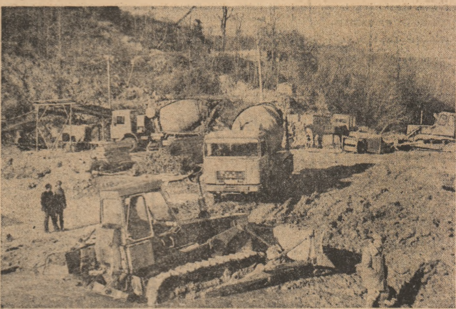
Pe șantierul microhidrocentralei „Zăbala 4 A” se lucrează la excavările pentru lacul de acumulare și la turnarea „prizei” de beton prin care apa va ajunge în turbinele de 0,65 MW.
